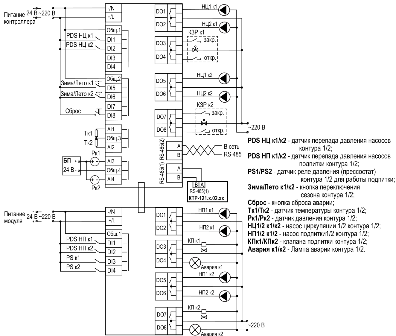
Рисунок 6.4 – Схема подключения KTR-121.03.20 для управления контурами ГВС и отопления с подпиткой
