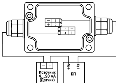
Рисунок 6 – «Сквозное» подключение
