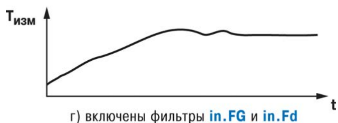
Рисунок Е.1 – Временные диаграммы работы Цифровых фильтров
