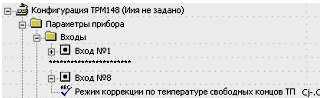
Рисунок 9.8 – Конфигуратор. КХС
