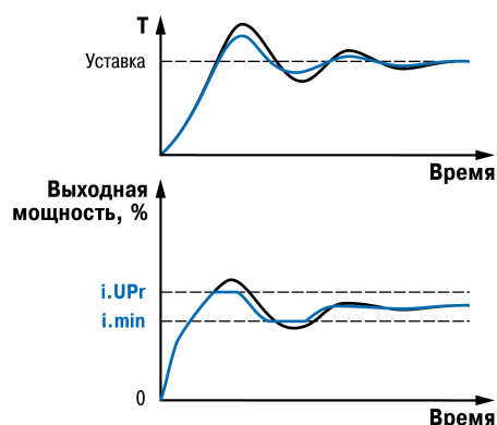
Рисунок 9.17 – ПИД-регулирование
