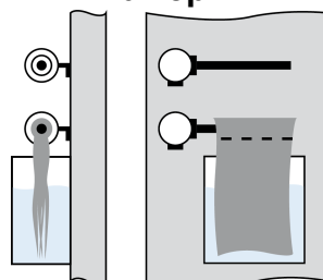
Рисунок Б.1 – Крепление датчиков температуры перпендикулярно стенке камеры
