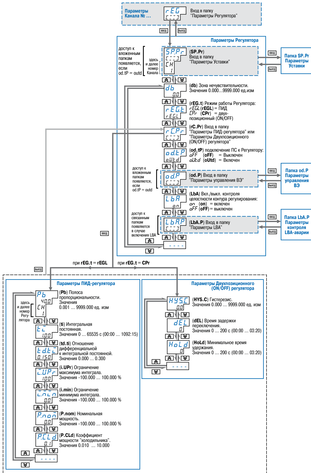
Рисунок 8.20 – Схема задания параметров Регуляторов
