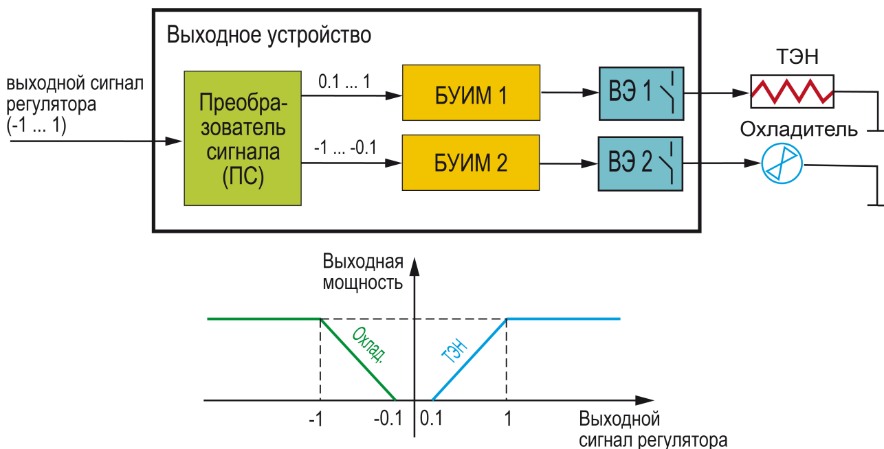
Рисунок 9.41 – Управление системой «нагреватель-холодильник»
