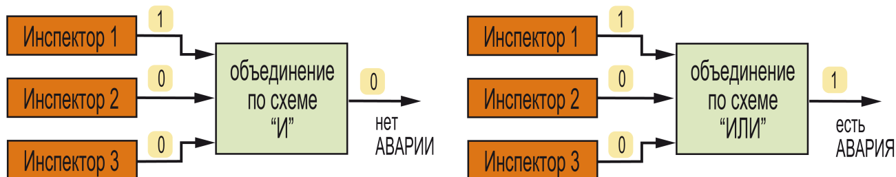
Рисунок 9.49 – Логика принятия решения об аварии
