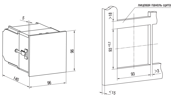
Рисунок 4.2 – Габаритные размеры корпуса Щ4
