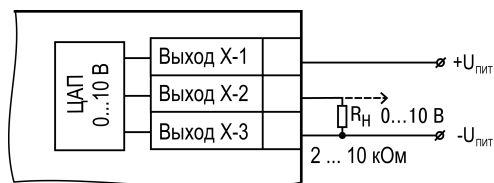
Рисунок 5.20 – Схема подключения нагрузки к ВУ типа У
