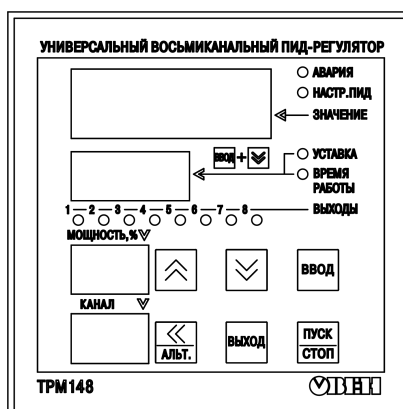
Рисунок 6.2 – Лицевая панель TRM148
