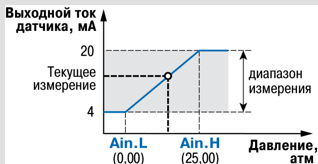
Рисунок 9.9 – Пример задания диапазона измерения активного датчика
