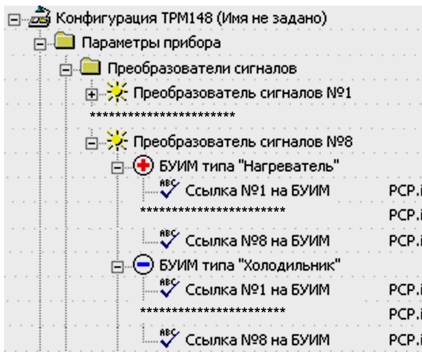
Рисунок 9.38 – Конфигуратор. Задание поддиапазонов
