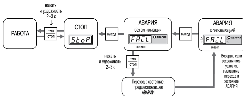
Рисунок 8.2 – Схема переключения состояний прибора
