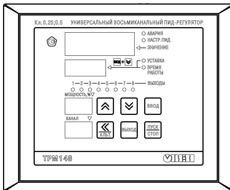
Рисунок 6.3 – Лицевая панель TRM148–Х.Щ7
