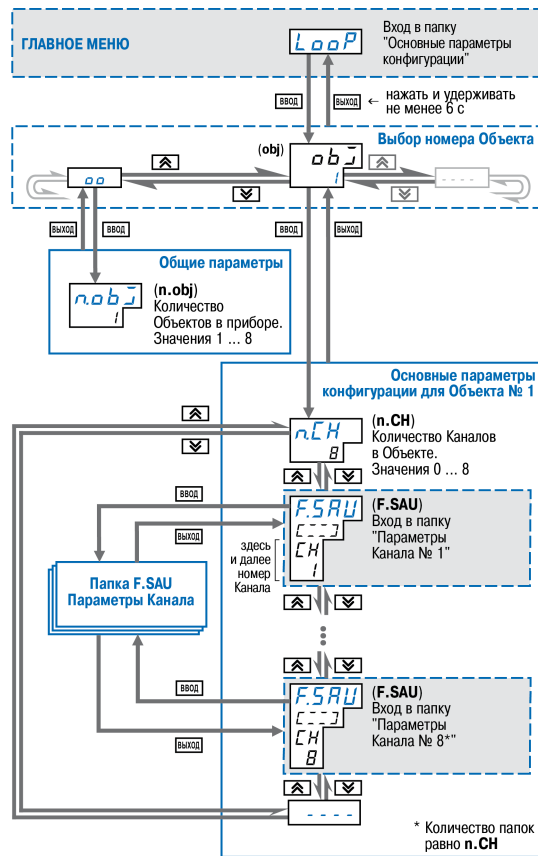
Рисунок 8.17 – Схема задания основных параметров конфигурации
