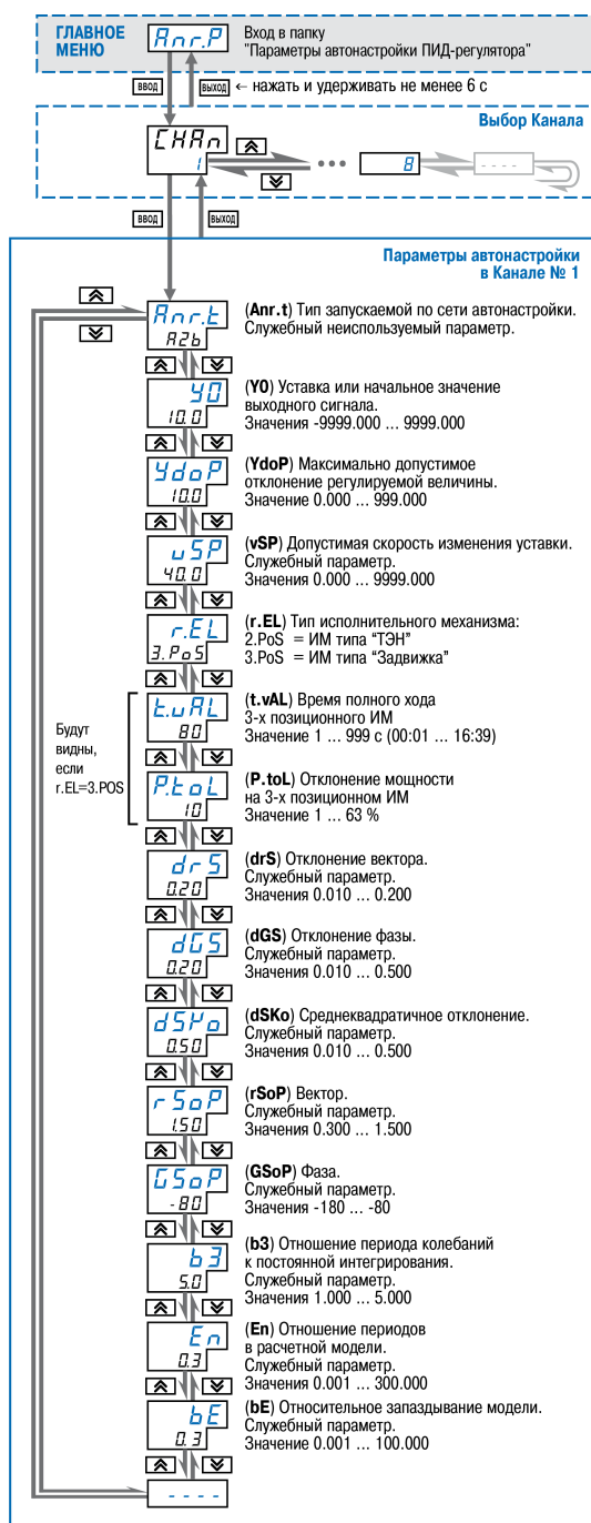
Рисунок 8.29 – Схема задания параметров Автонастройки ПИД-регулятора
