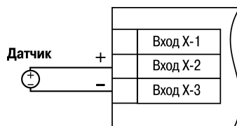
Рисунок 5.7 – Схема подключения активного датчика с выходом в виде напряжения -50...50 В или 0...1 В
