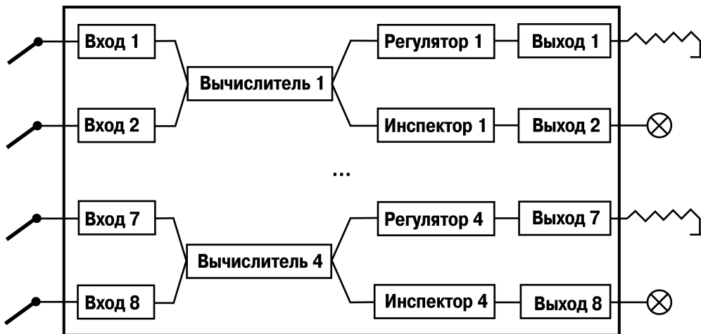
Рисунок 7.9 – Принципиальная схема модификации 4
