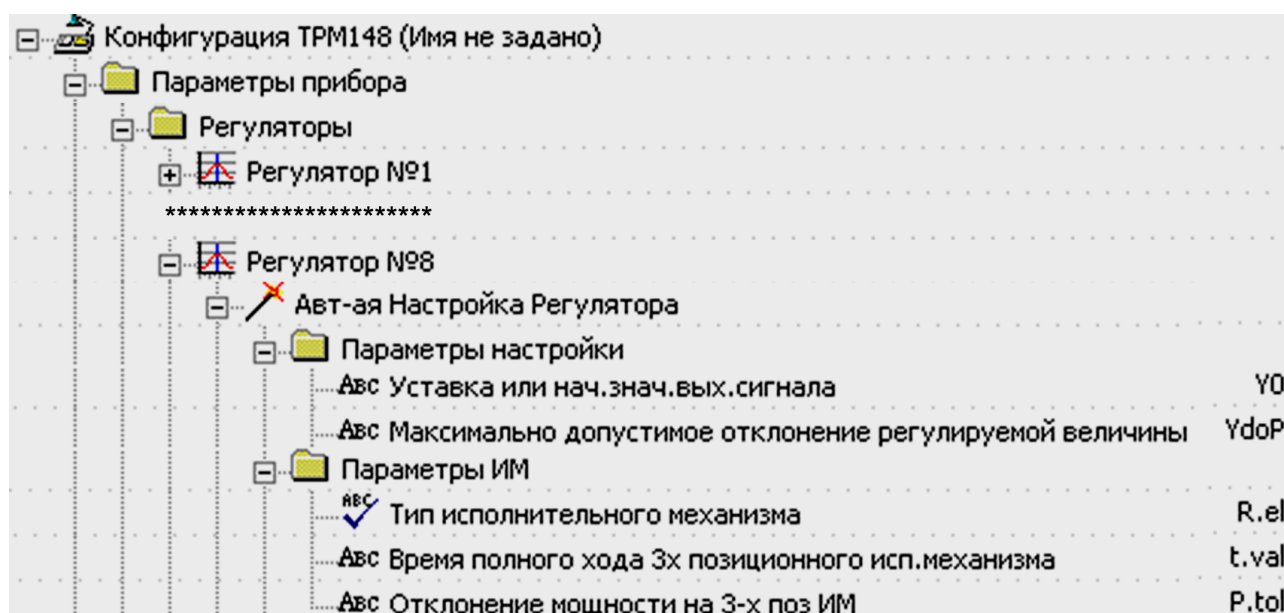
Рисунок 9.19 – Конфигуратор. Задание параметров ИМ
