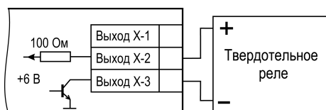
Рисунок 5.17 – Схема подключения нагрузки к ВУ типа Т
