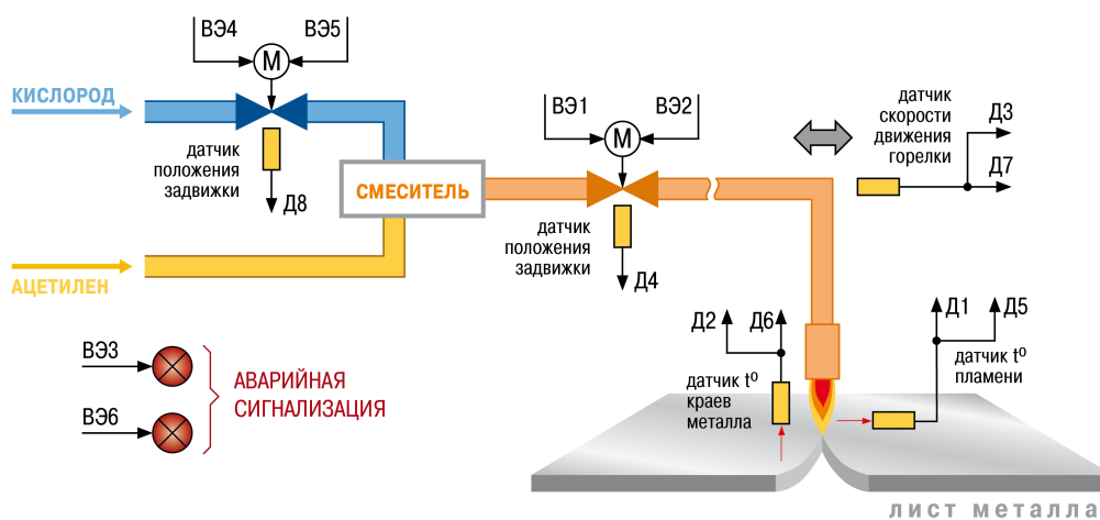
Рисунок 7.15 – Использование 8-канального регулятора TRM148 6-ой модификации в производственной автоматизированной установке резания листов из металлических сплавов
