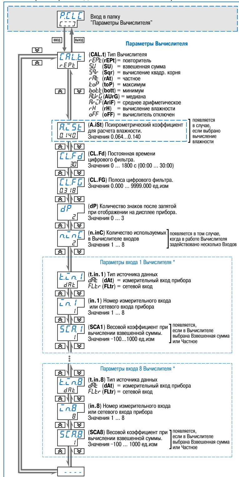
Рисунок 8.19 – Схема задания параметров Вычислителей
