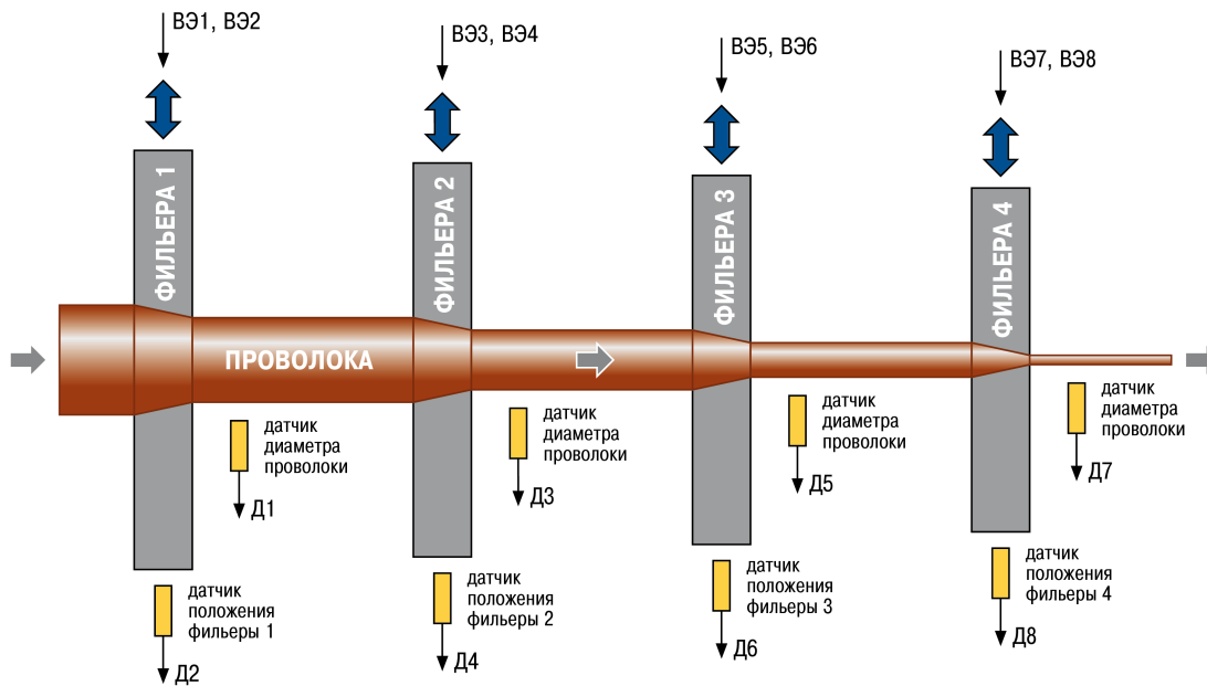
Рисунок 7.8 – Использование 8-канального регулятора ТРМ148 3-ой модификации в управляемой автоматизированной системе из четырех фильер для получения проволоки
