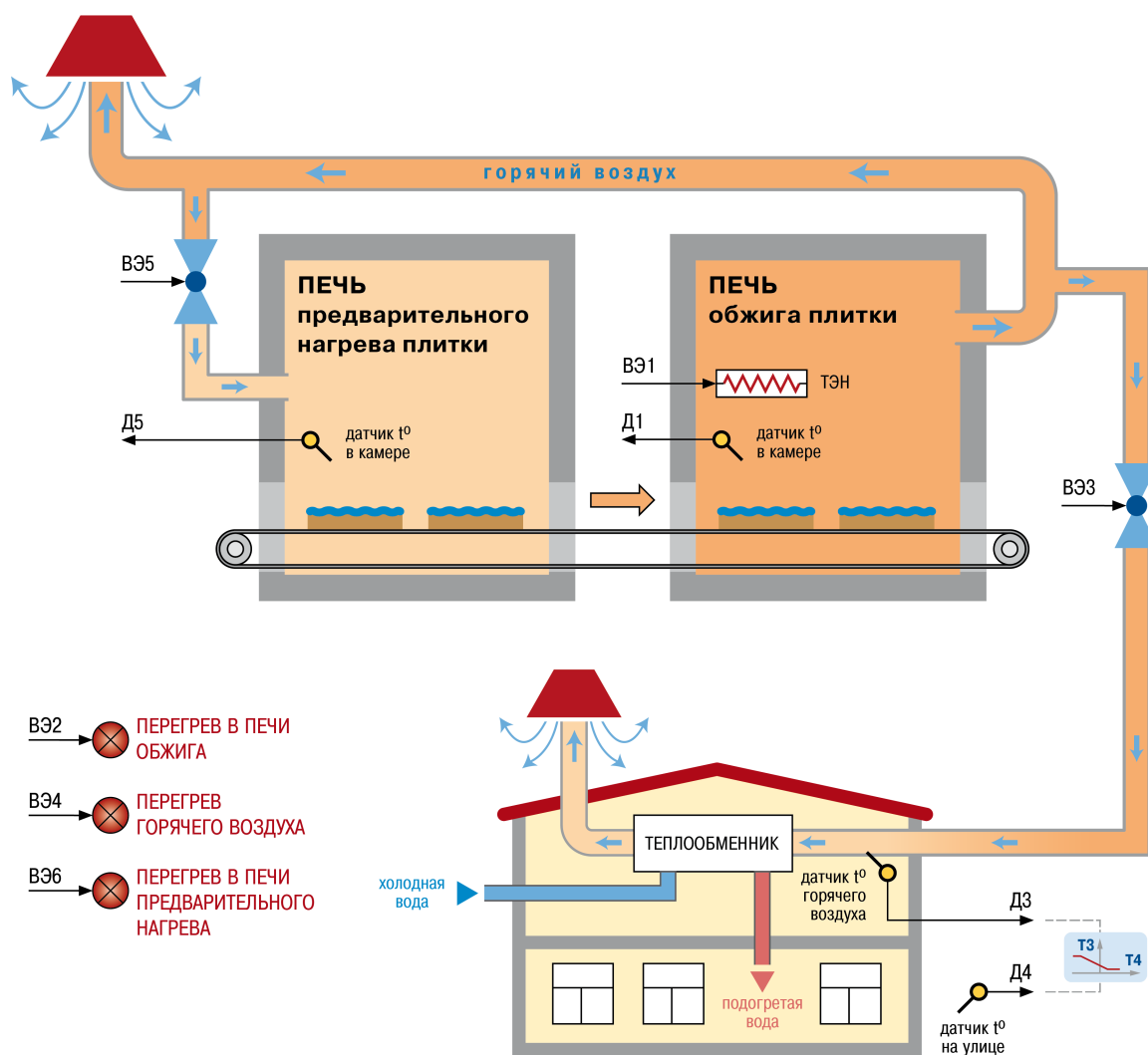
Рисунок 7.13 – Использование 8-канального регулятора TRM148 5-ой модификации в системе термообработки (обжига) керамической плитки
