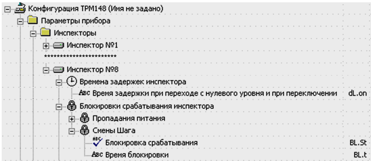
Рисунок 9.55 – Конфигуратор. Блокировка первого срабатывания
