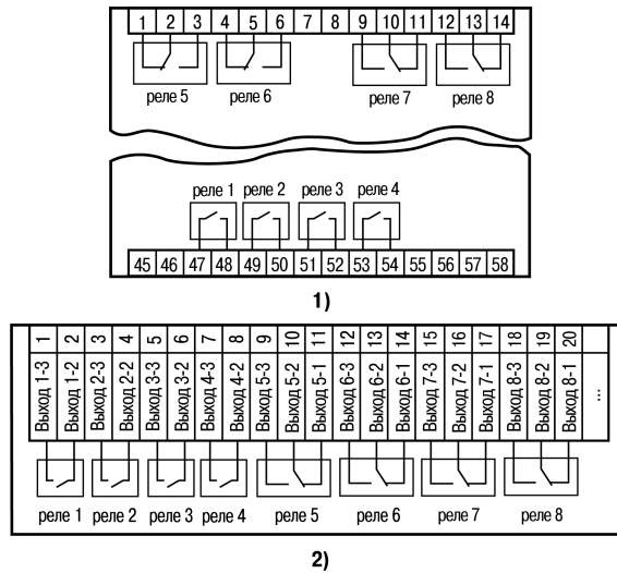
Рисунок 5.11 – Схема подключения электромагнитных реле прибора: 1) в корпусе Щ4, 2) в корпусе Щ7
