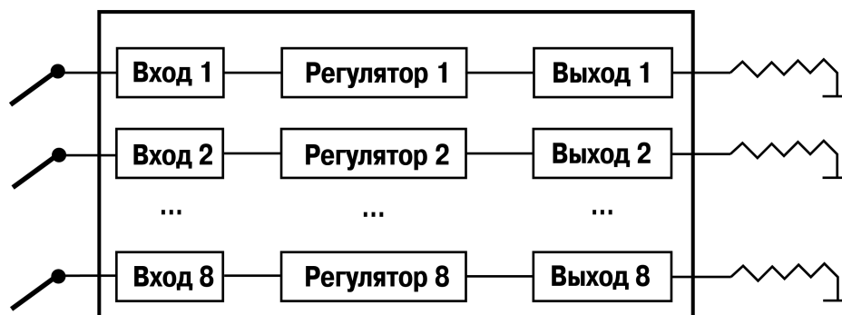
Рисунок 7.1 – Принципиальная схема модификации 1
