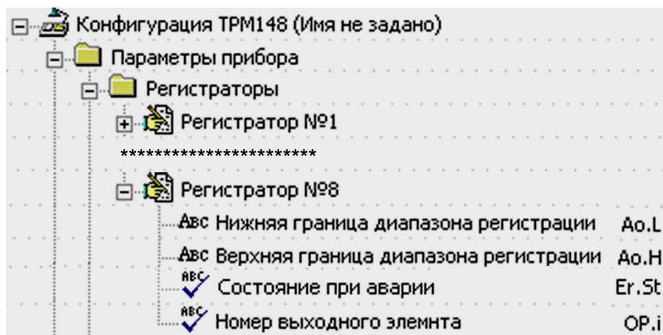
Рисунок 9.58 – Конфигуратор. Параметры Регистратора
