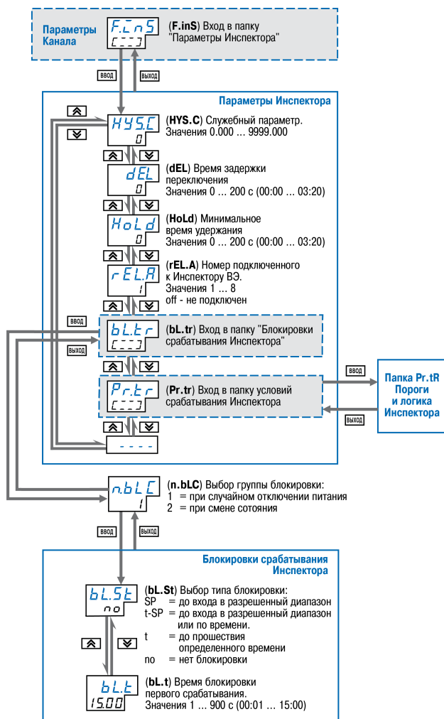
Рисунок 8.26 – Схема задания параметров Инспектора
